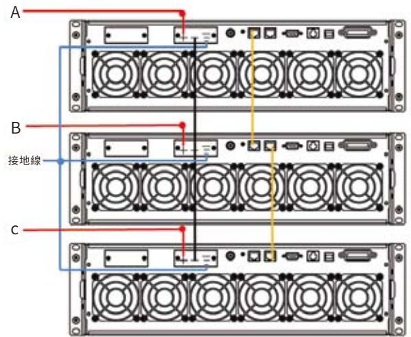
三角形接法
