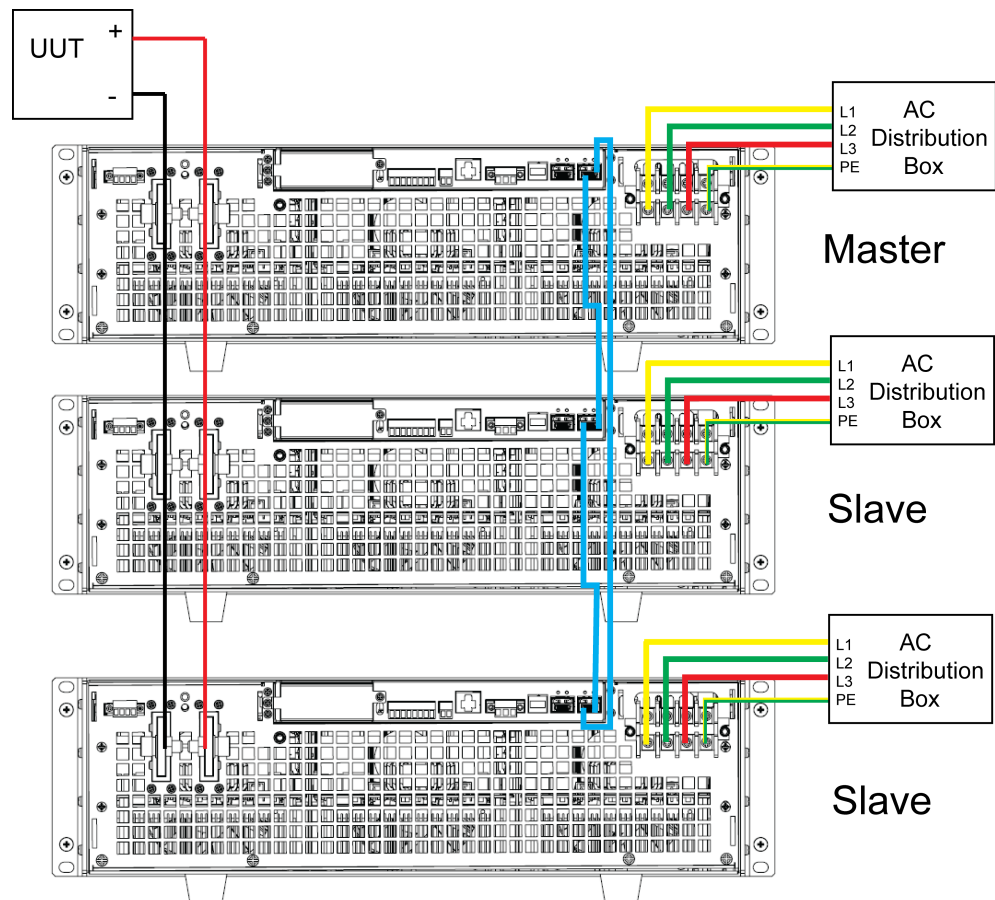
圖 5-1 線路連接圖
