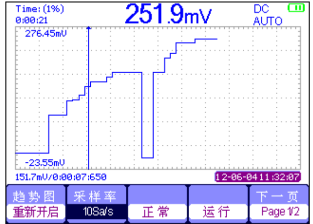
万用表趋势图
