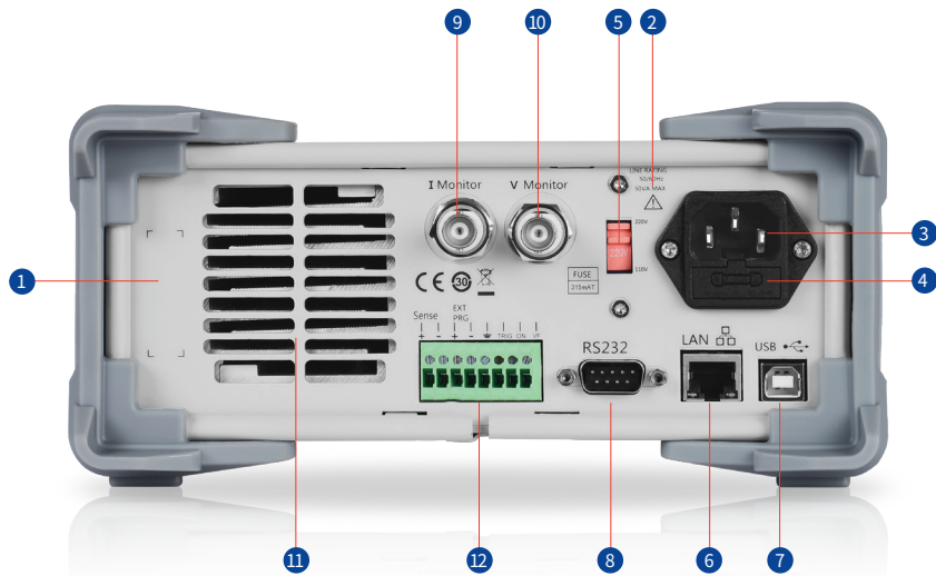
图 2 SDL1000X 后面板
