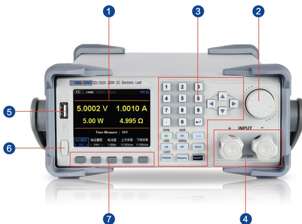
图 1 SDL1020X 前面板
