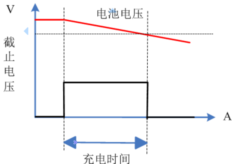
图 2-37 Battery 测试功能
