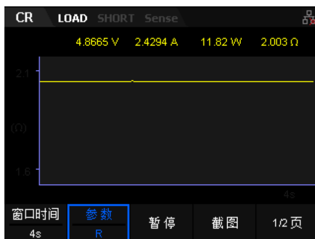
图 2-10 CR 模式波形显示界面
