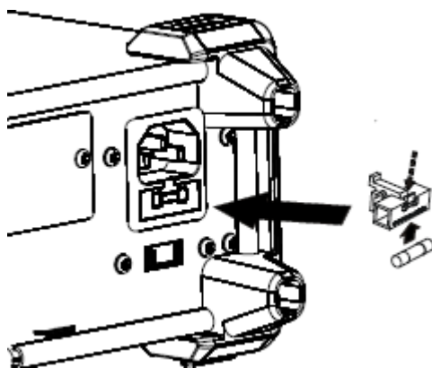
图 1-7 更换保险丝
