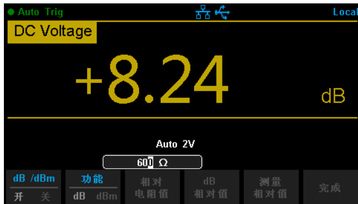
图 2- 47 运算设置界面
