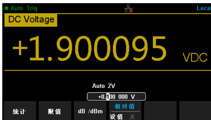
图 2- 48 相对运算设置界面
