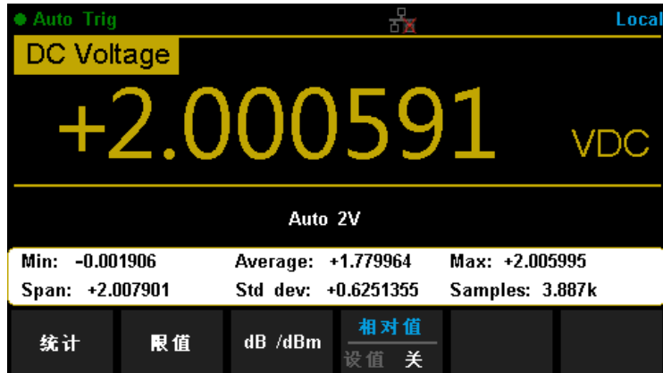
图 2-44 统计运算菜单界面
