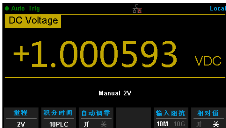
图 2-5 设置自动调零
