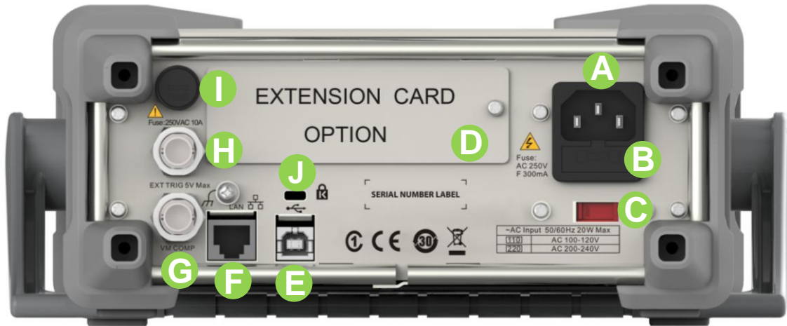
图 1-6 后面板示意图
