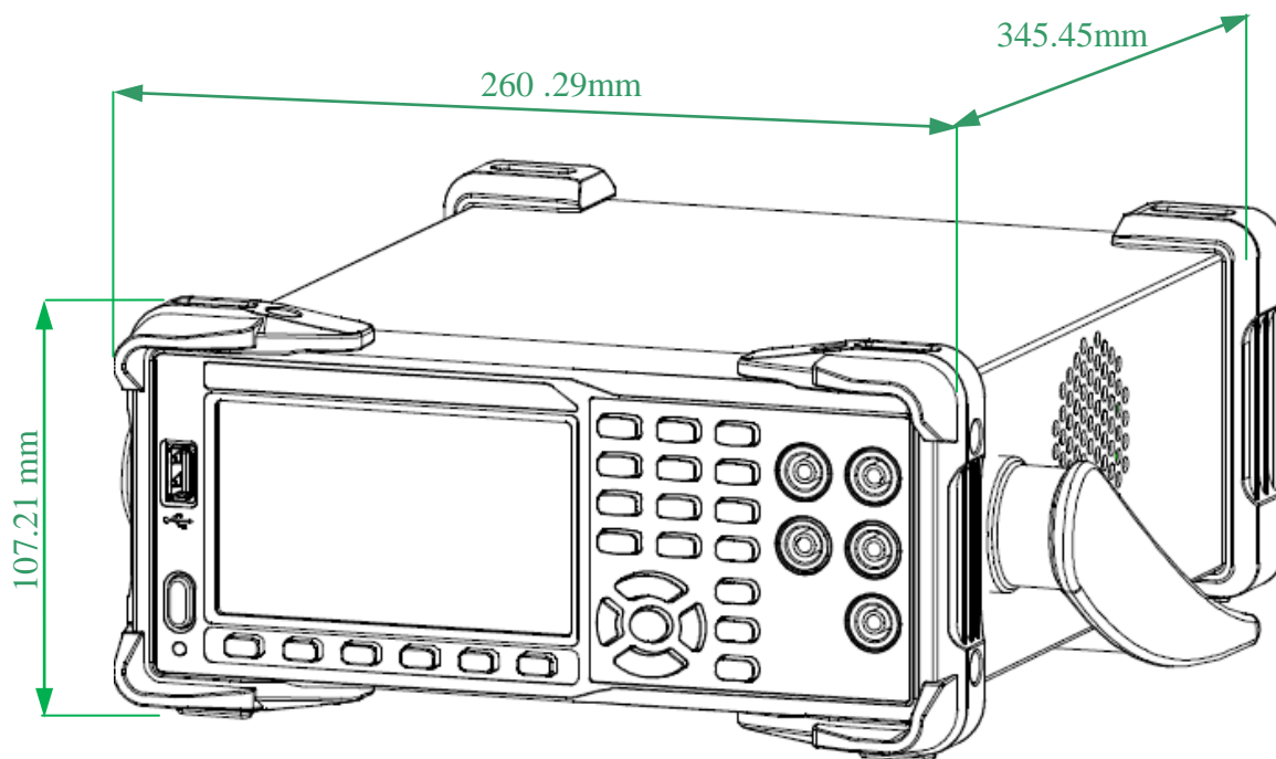
图 1-4 外观尺寸
