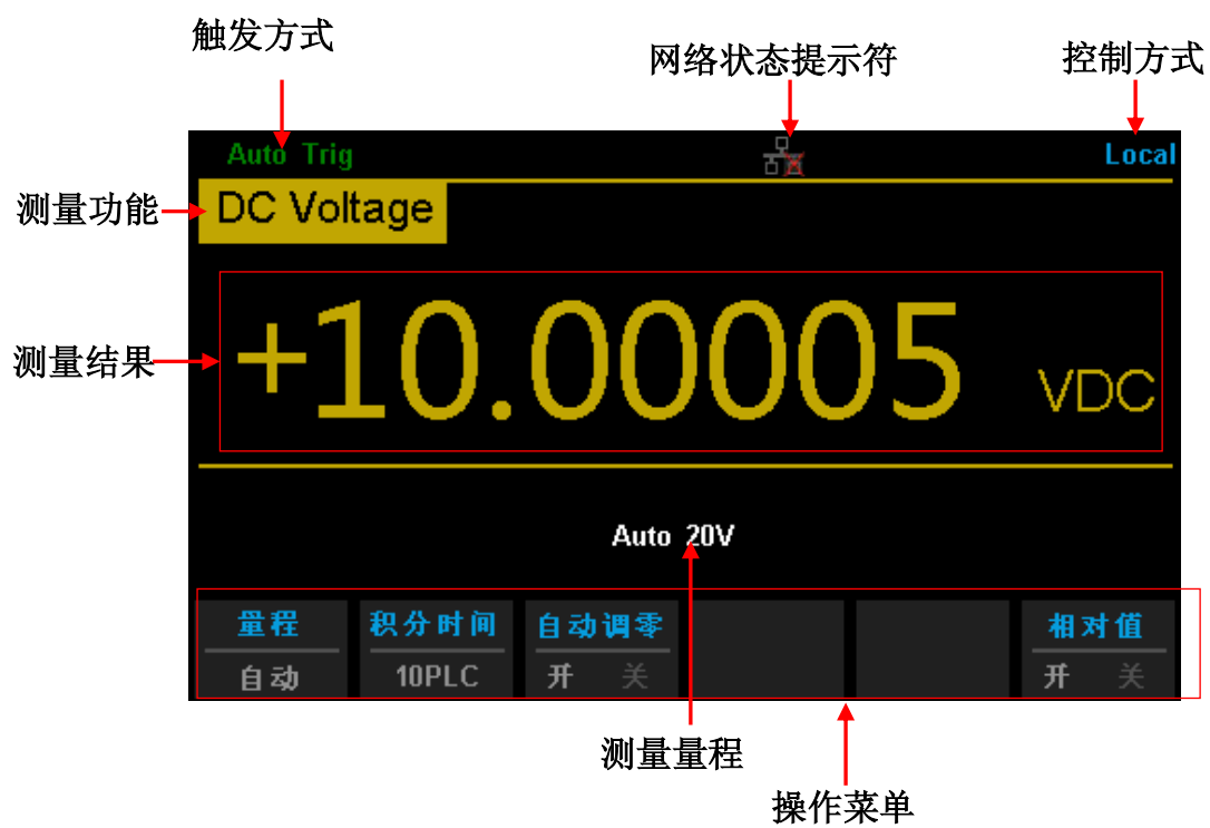
图 1-8 用户界面
