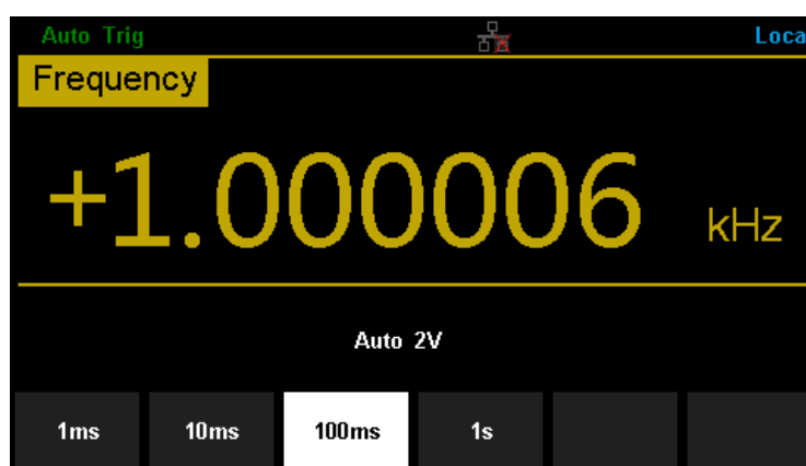
图 2-9 设置闸门时间
