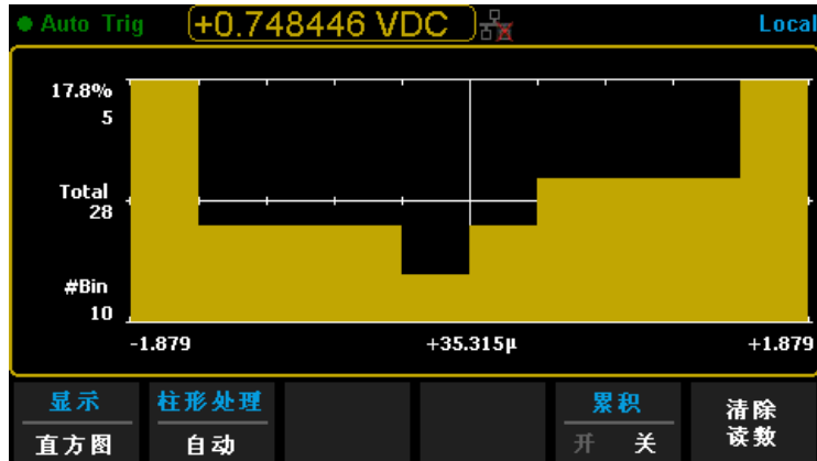
图 2- 52 直方图显示模式
