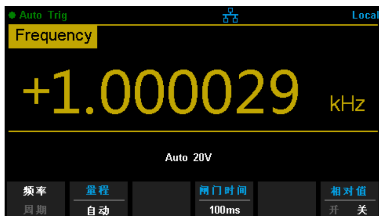
图 2-17 频率测量界面
