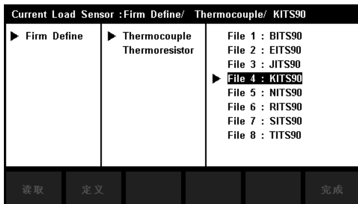
图 2-22 加载配置文件界面
