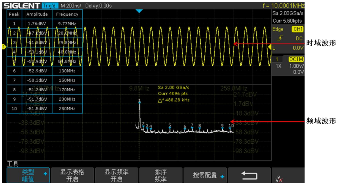
图 91 FFT 波形
