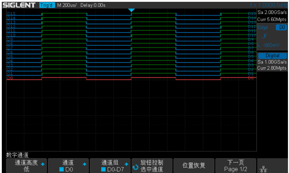
图 126 通道高度选择低
