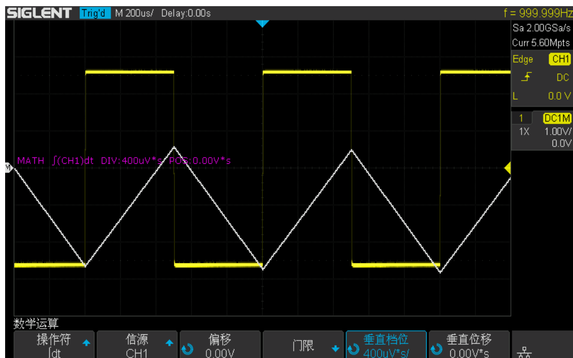
图 93 无 DC 偏移校正（积分运算）
