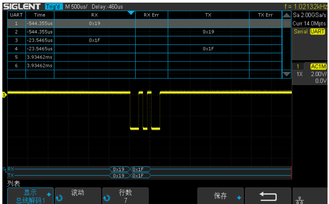
图 66 UART 解码图
