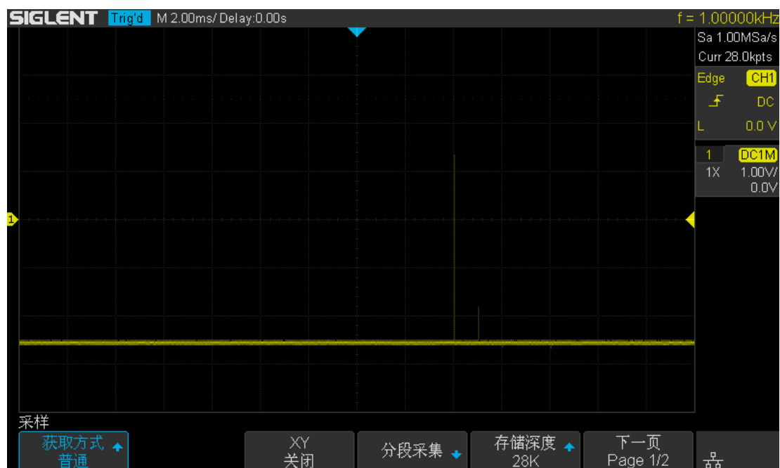
图 26 带窄脉宽的方波（普通模式）
