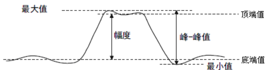
图 99 电压参数示意图
