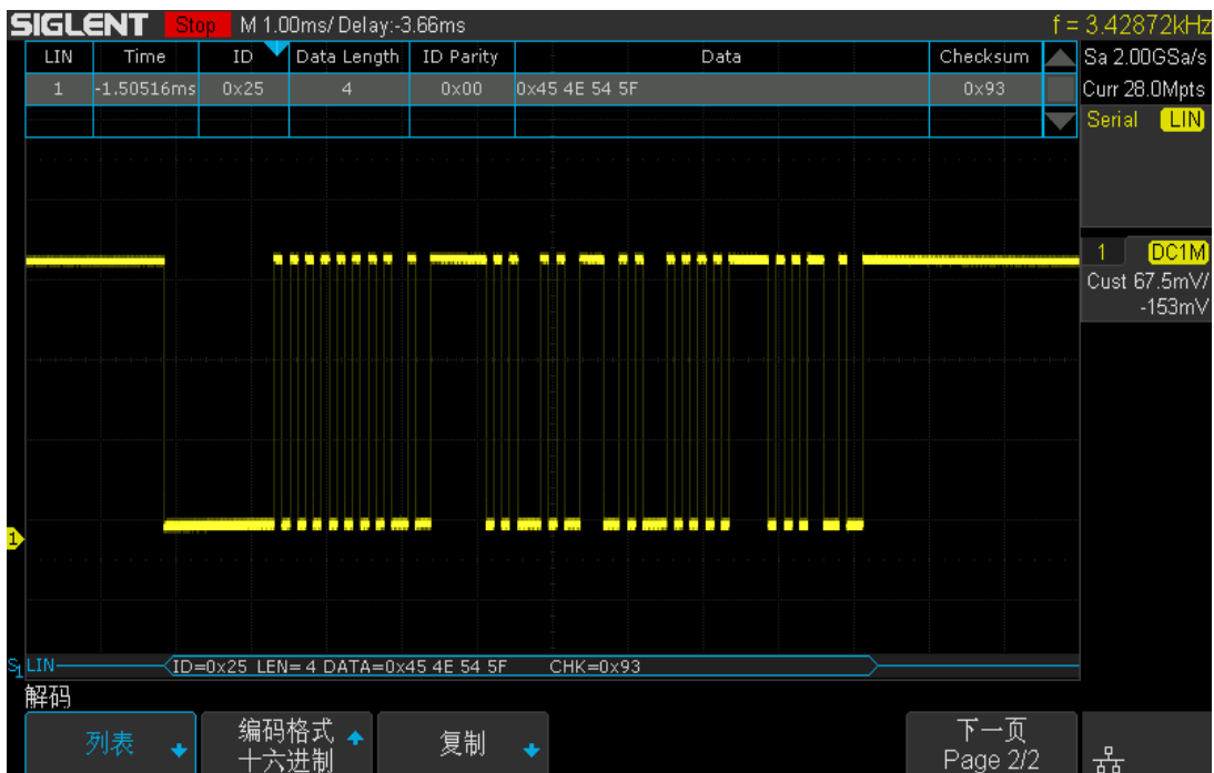
图 77 LIN 解码
