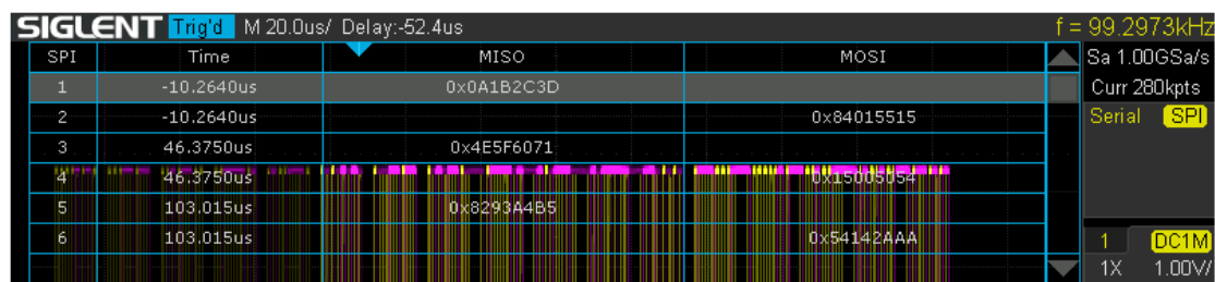
图 59 SPI 解码列表显示
