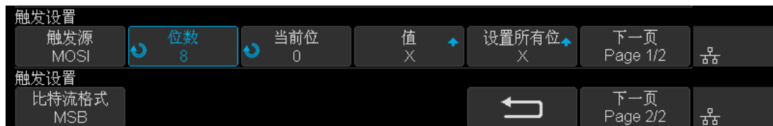
图 56 SPI 触发设置菜单
