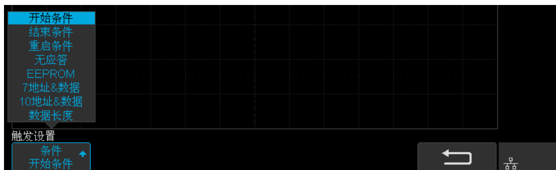
图 47 I2C 触发条件
