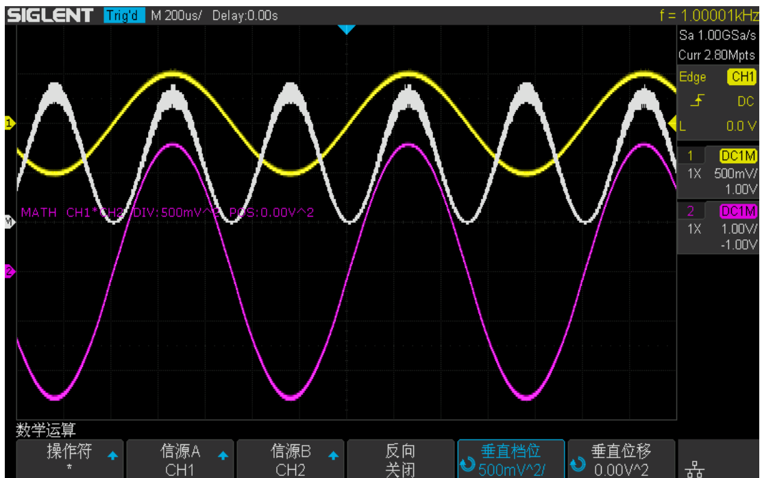
图 82 通道 1 波形乘以通道 2 波形
