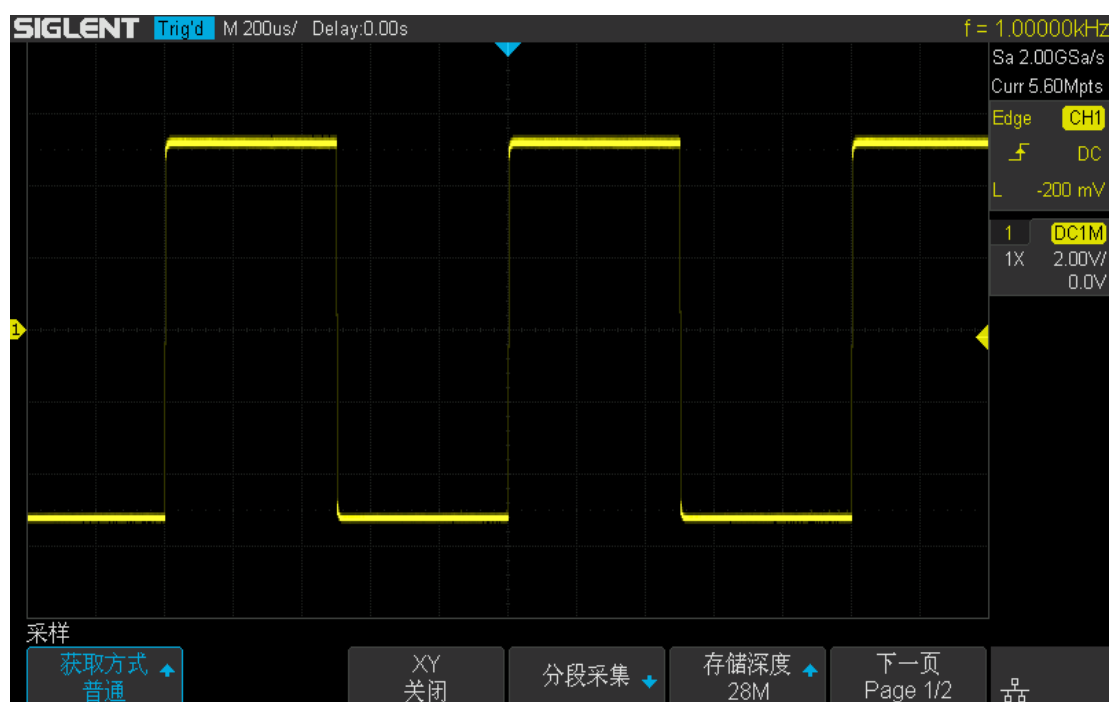
图 28 未平均时的波形（显示波形上的随机噪声）
