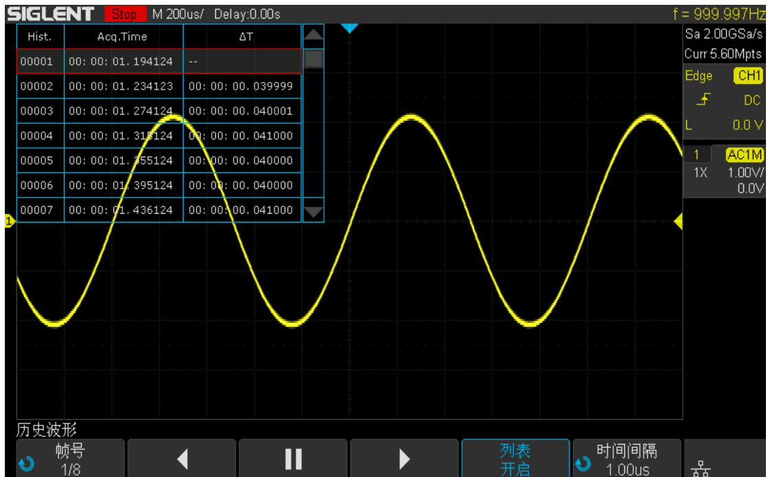
图 107 历史波形功能菜单
