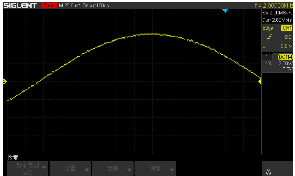
图 15 扩展后的毛刺正弦波
