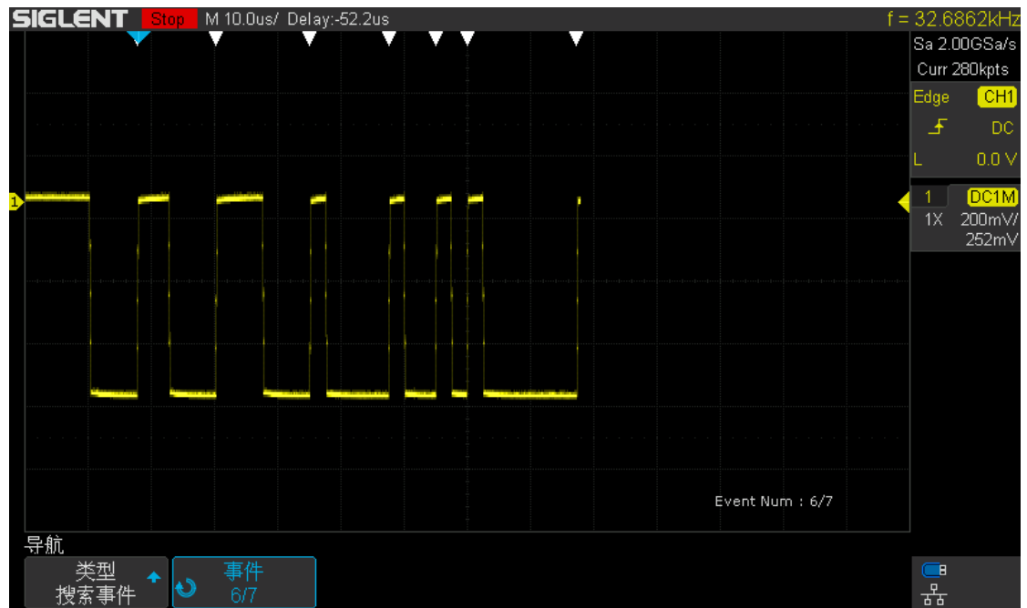
图 113 搜索事件导航
