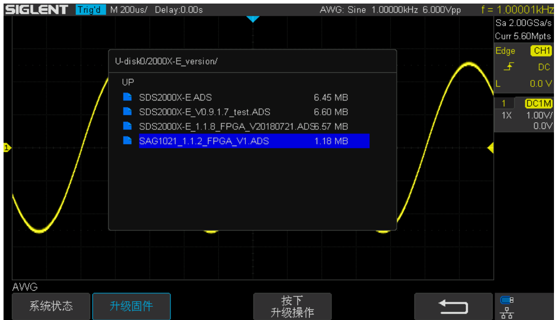
图 153 AWG 固件升级界面
