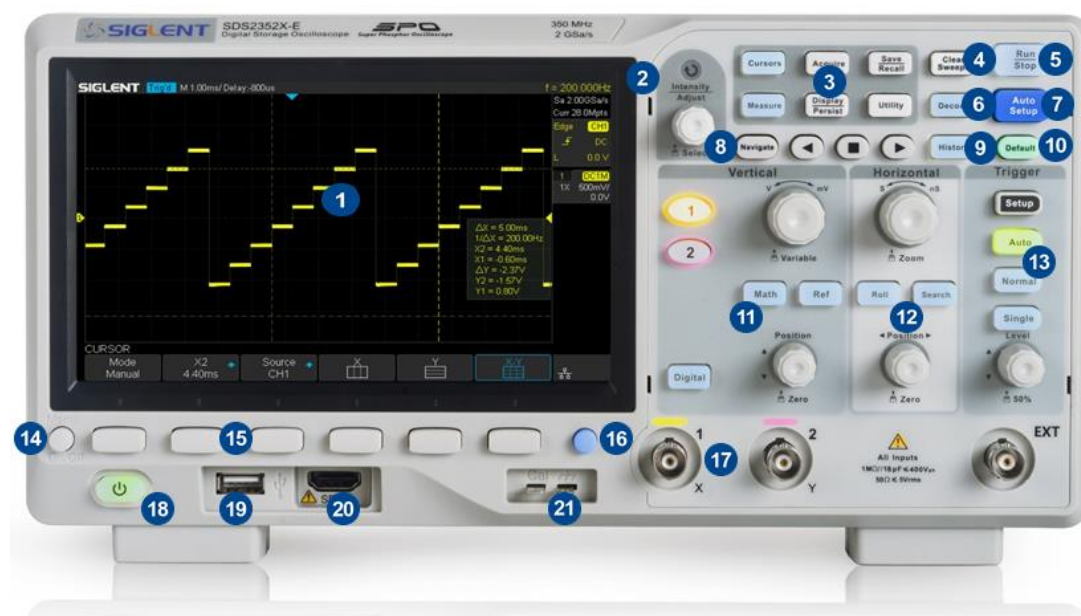
图 6 前面板总览
