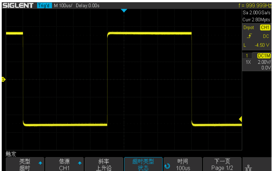
图 42 “状态”超时触发
