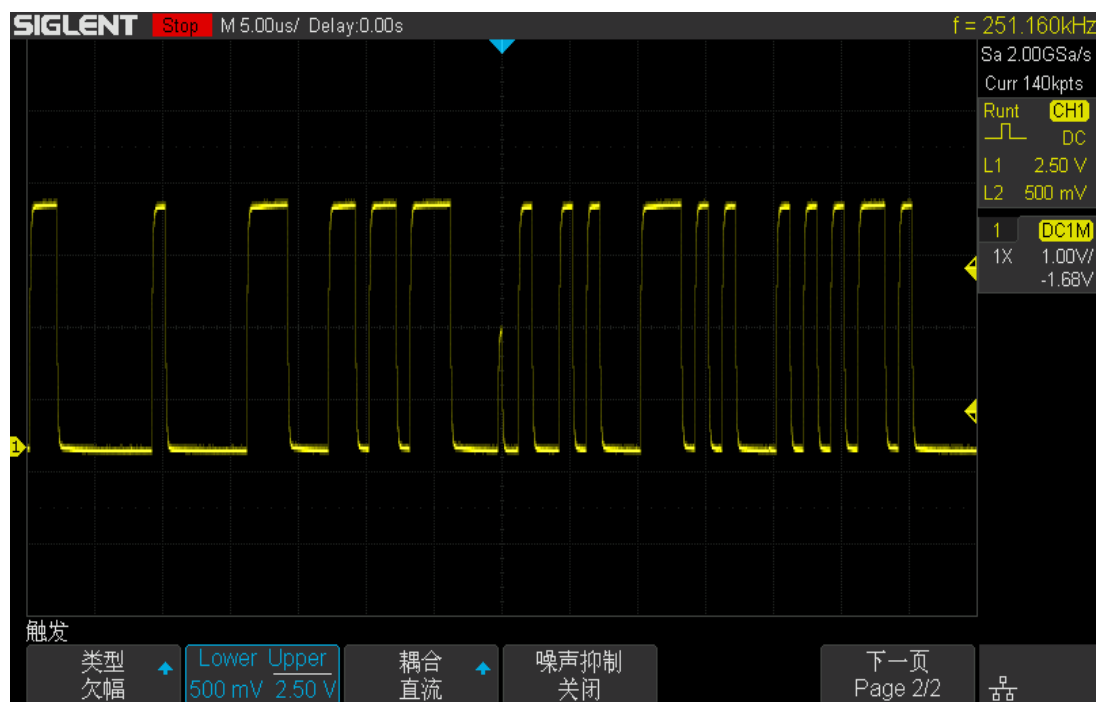
图 43 欠幅脉冲触发
