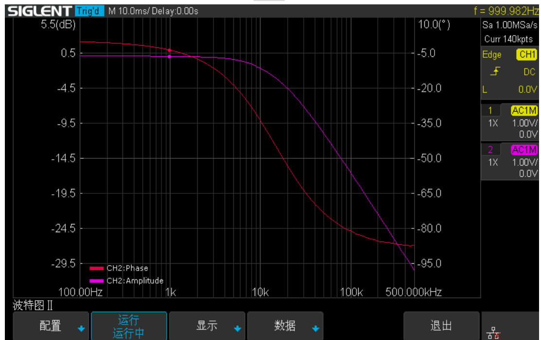
图 170 可变幅值下波特图扫描曲线
