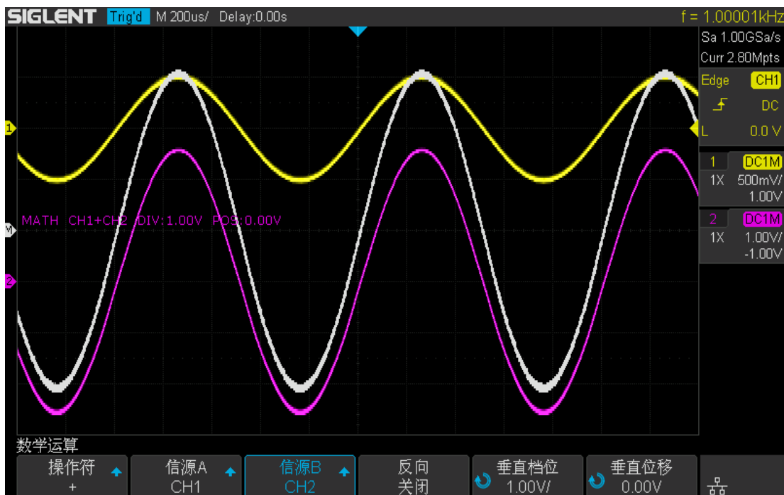
图 81 通道 1 波形加通道 2 波形
