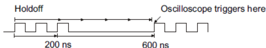
图 31 设置触发释抑时间
