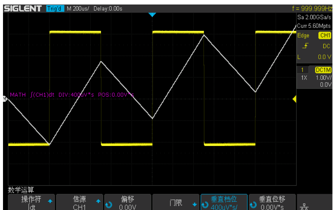
图 94 有 DC 偏移校正（积分运算）
