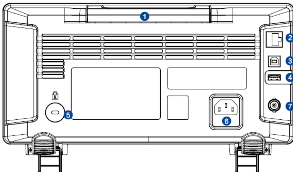
图 7 后面板总览
