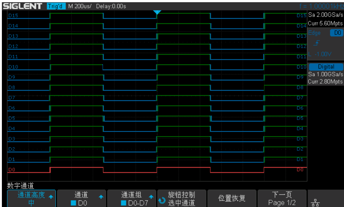
图 125 通道高度选择中
