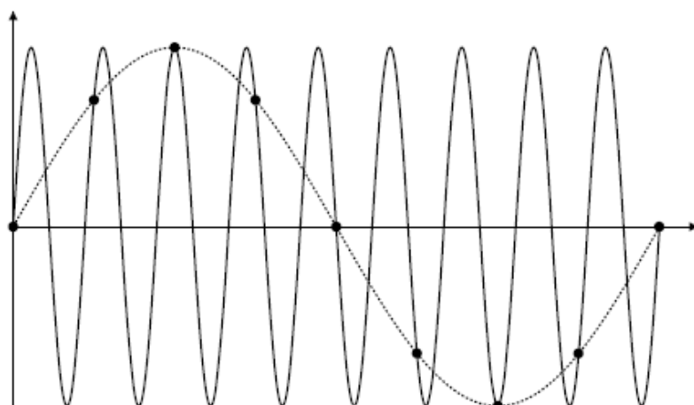
图 19 采样混叠
