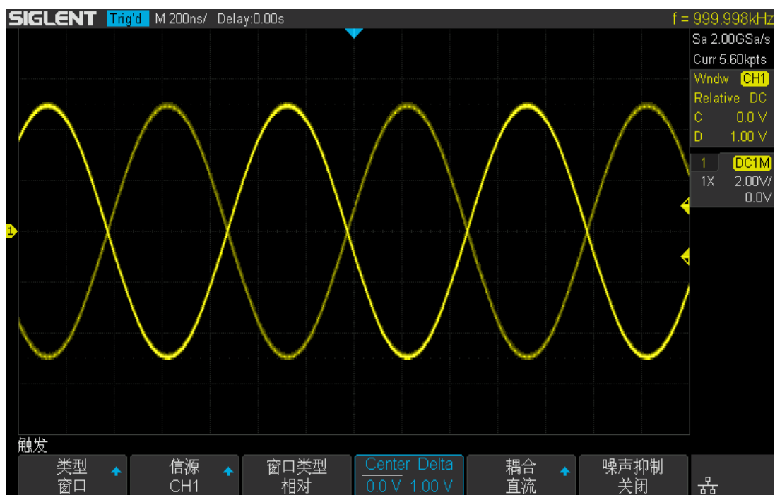
图 39 “相对”窗口触发
