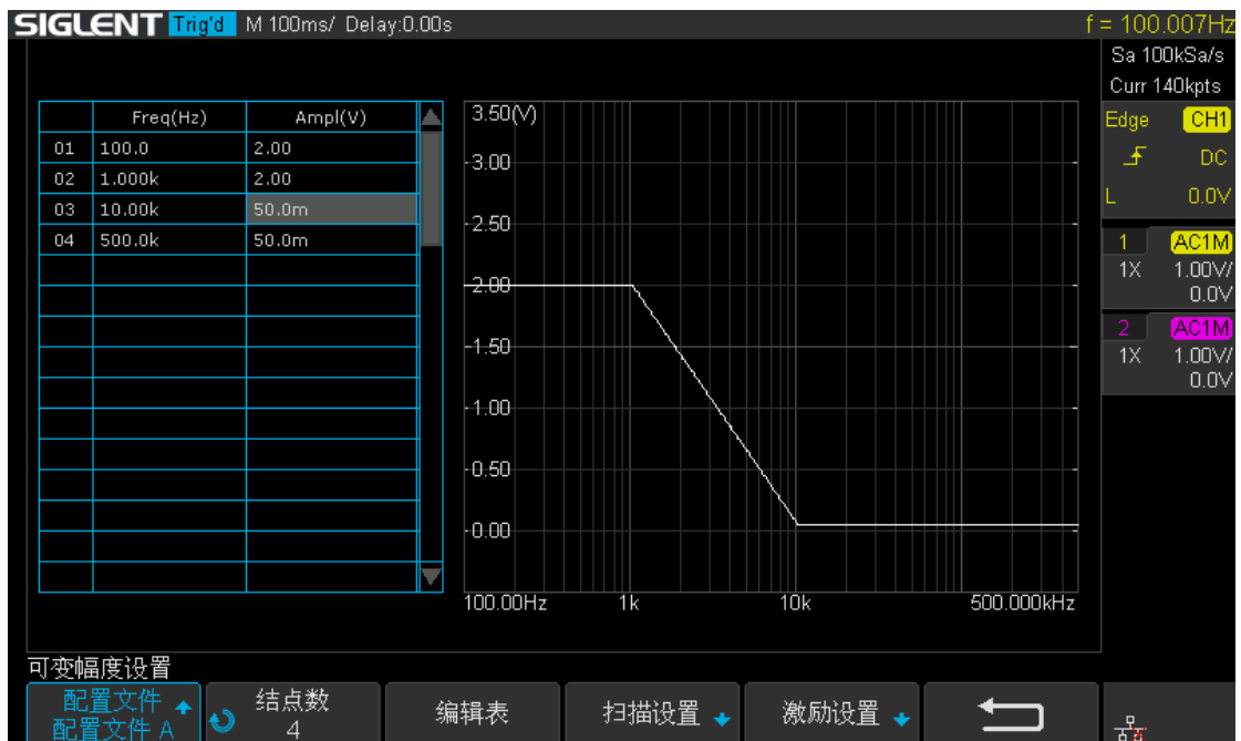
图 168 可变幅度的编辑表菜单
