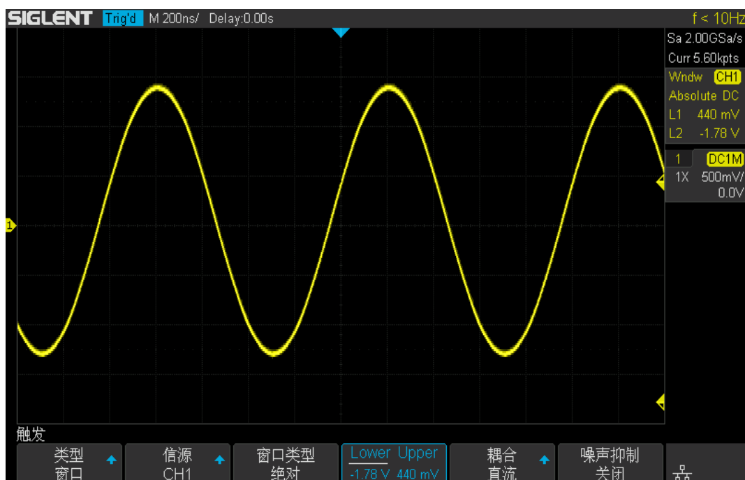
图 38 “绝对”窗口触发
