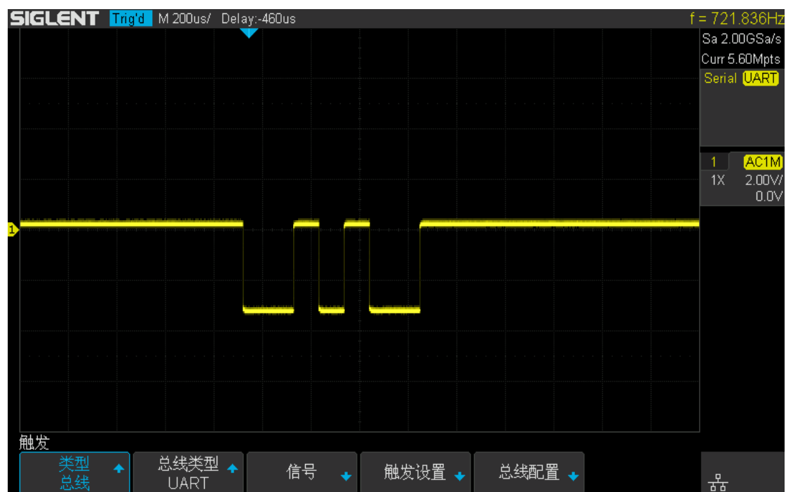
图 64 UART 触发
