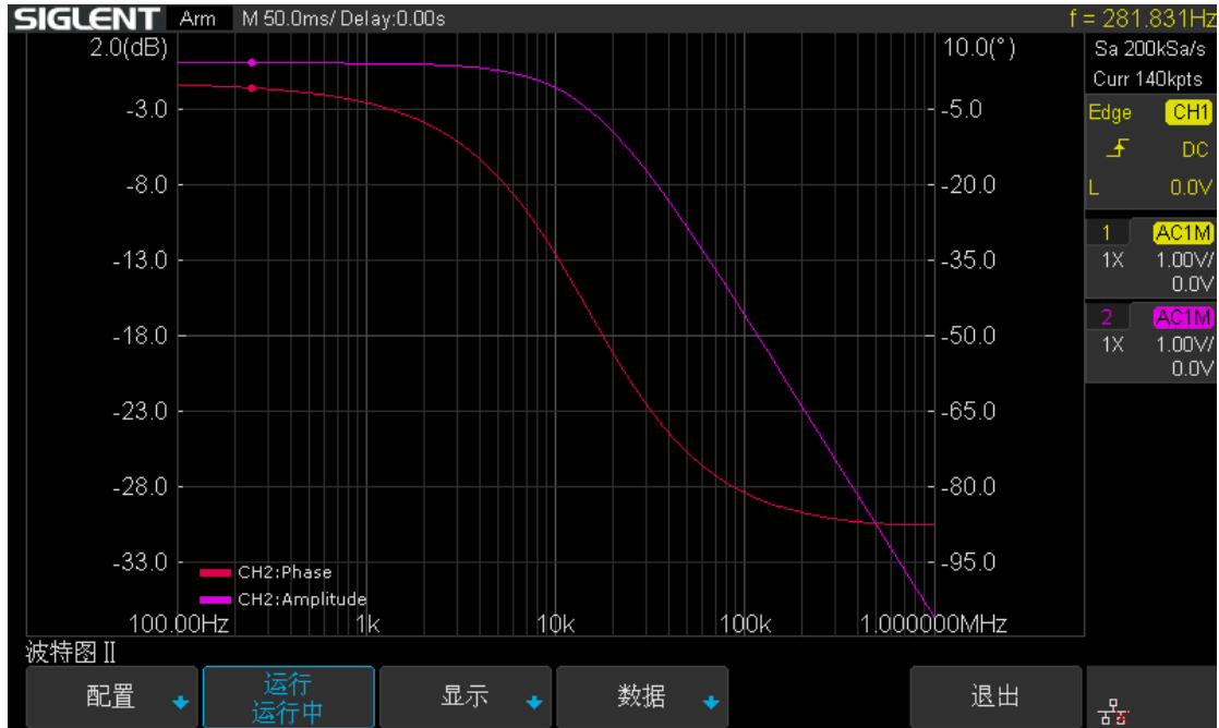
图 165 恒定幅值下波特图扫描曲线
