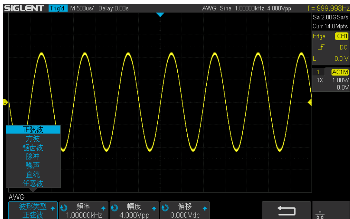
图 149 基本波形选择
