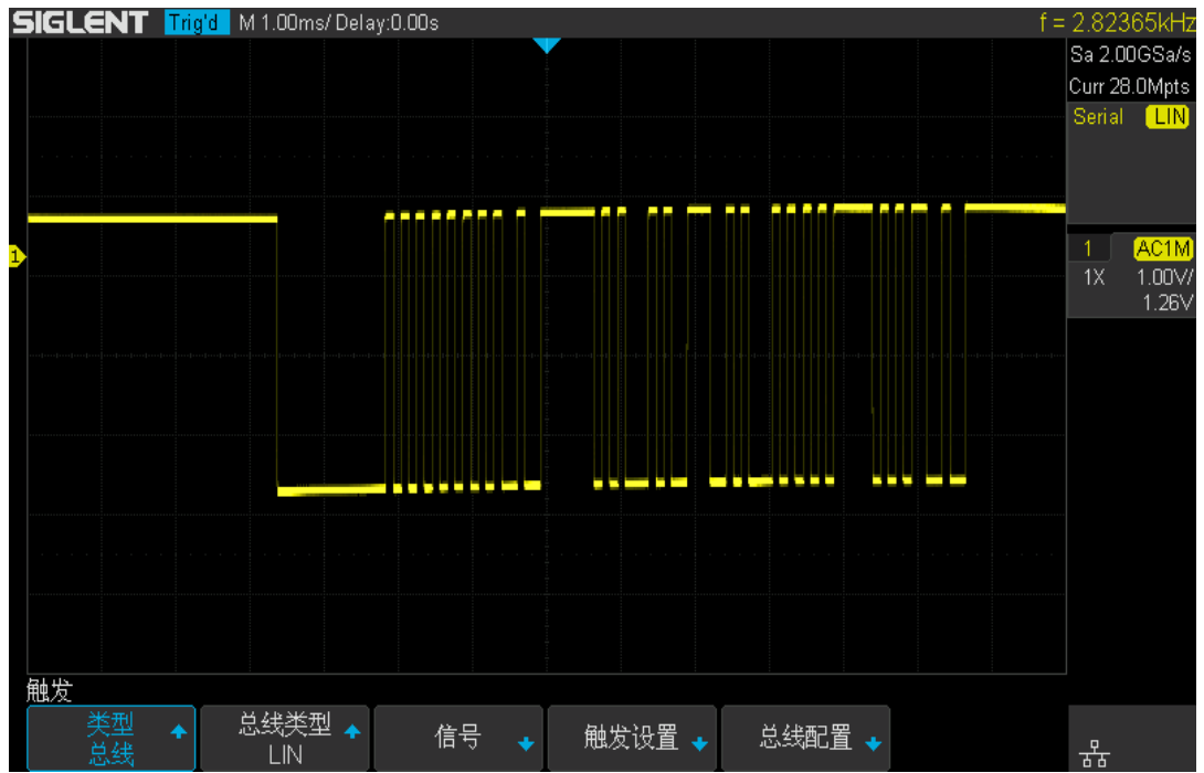
图 76 LIN 触发
