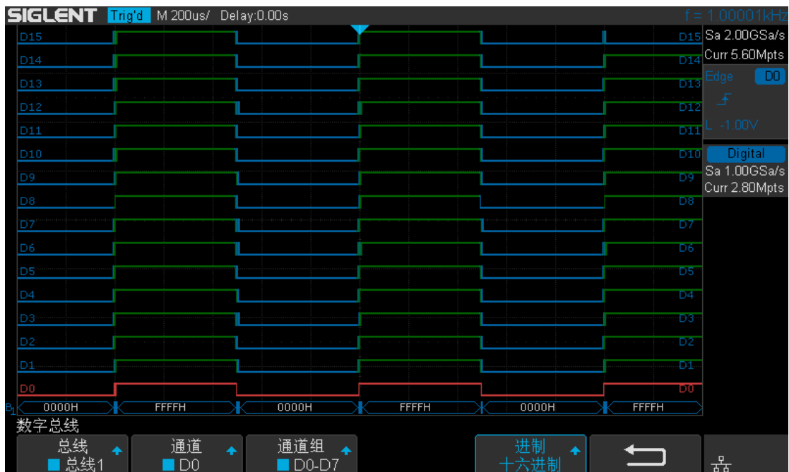
图 129 数字总线
