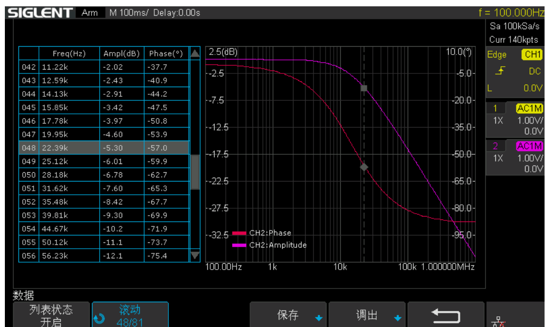
图 159 波特图列表
