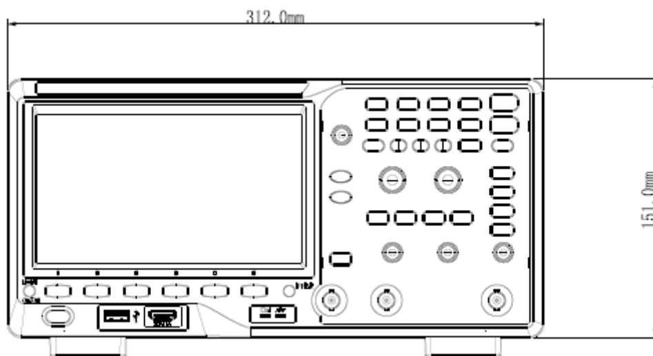
图 1 正视图
