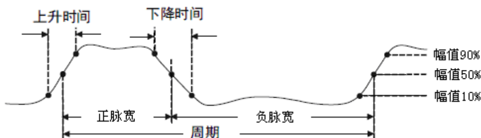
图 102 时间参数示意图
