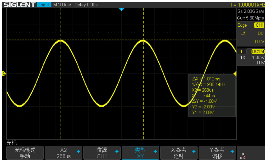
图 96 光标测量
