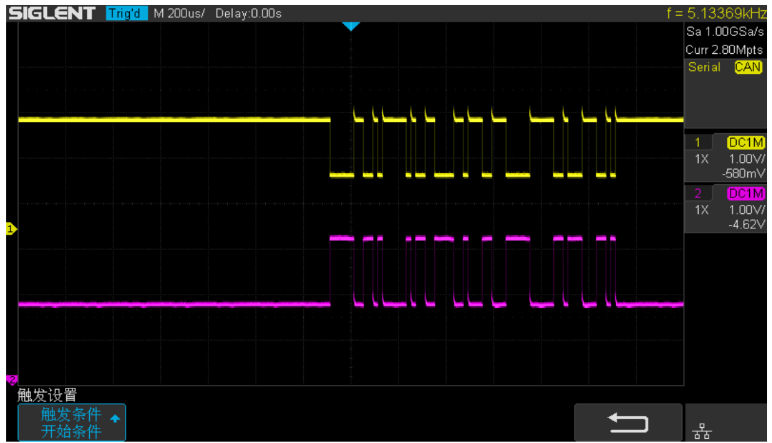
图 71 CAN 触发
