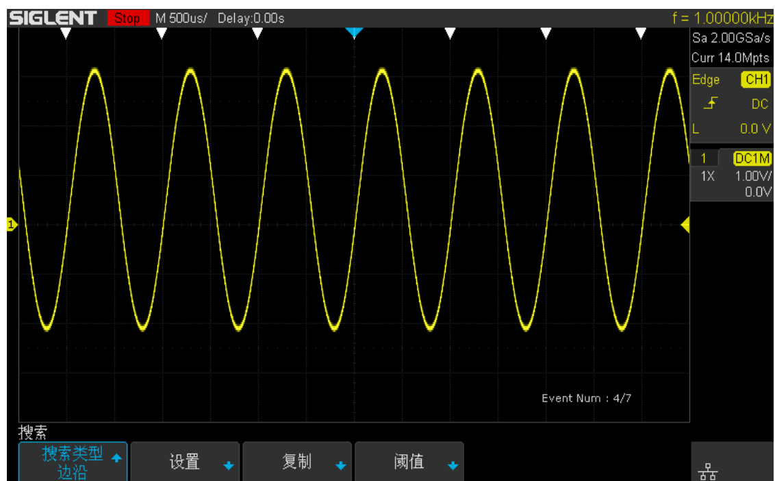
图 110 停止状态下搜索结果显示
