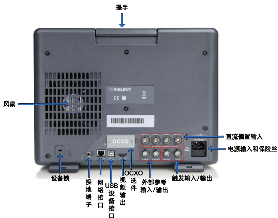
图 8-1 后面板功能划分
