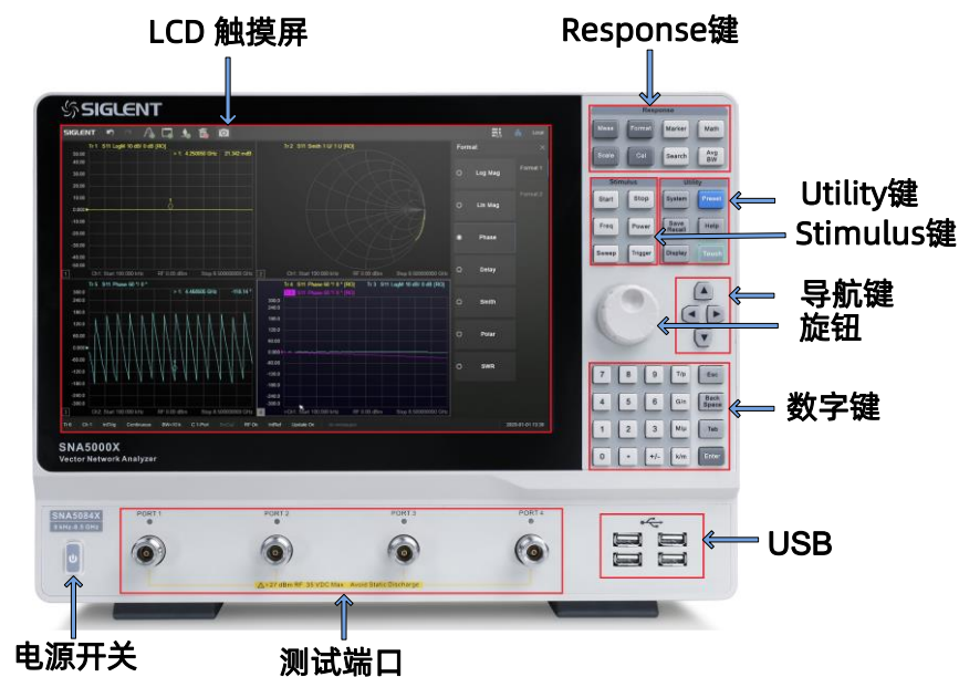
图 7-1 前面板
