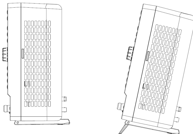
图 6-1 支撑脚调节示意图
