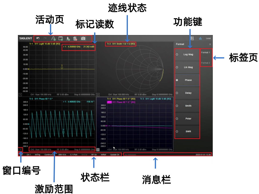
图 9-1 用户界面
