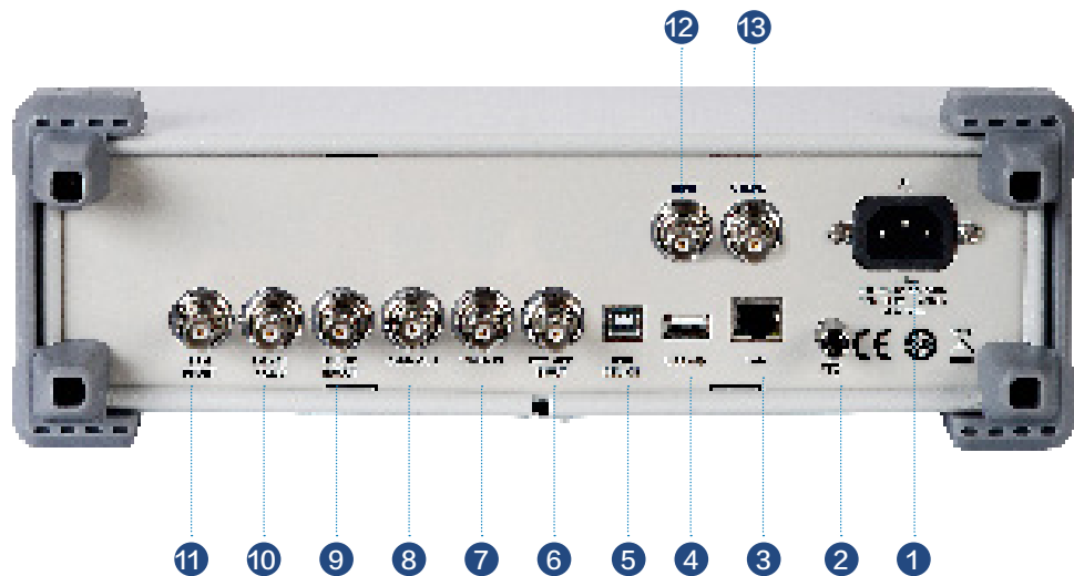
图 1-7 后面板
