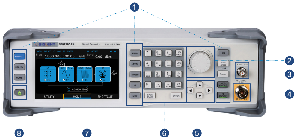
图 1-4 前面板
